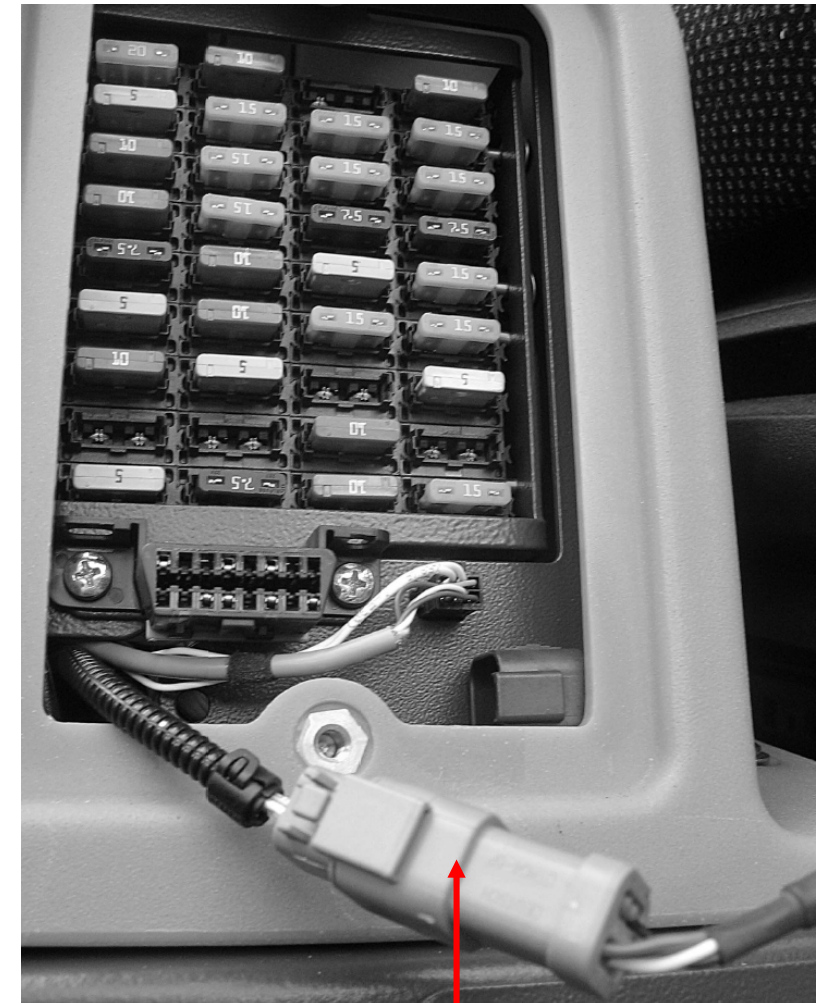
X59 mit angeschlossenem Diagnosekabel zum Yanmar Interface X59 with connected diagnosis cable to Yanmar- Interface
